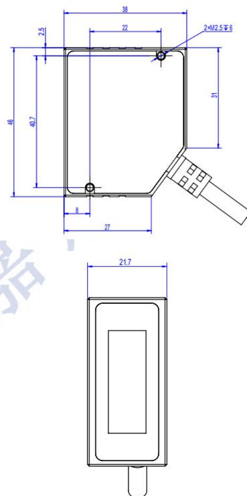
尺寸图
